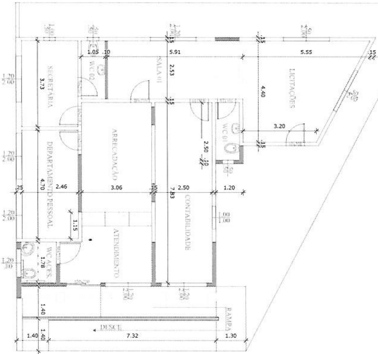
01 - Planta Baixa
